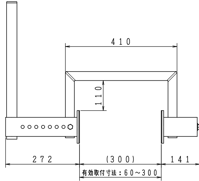
【取付寸法 300 mm の場合】
