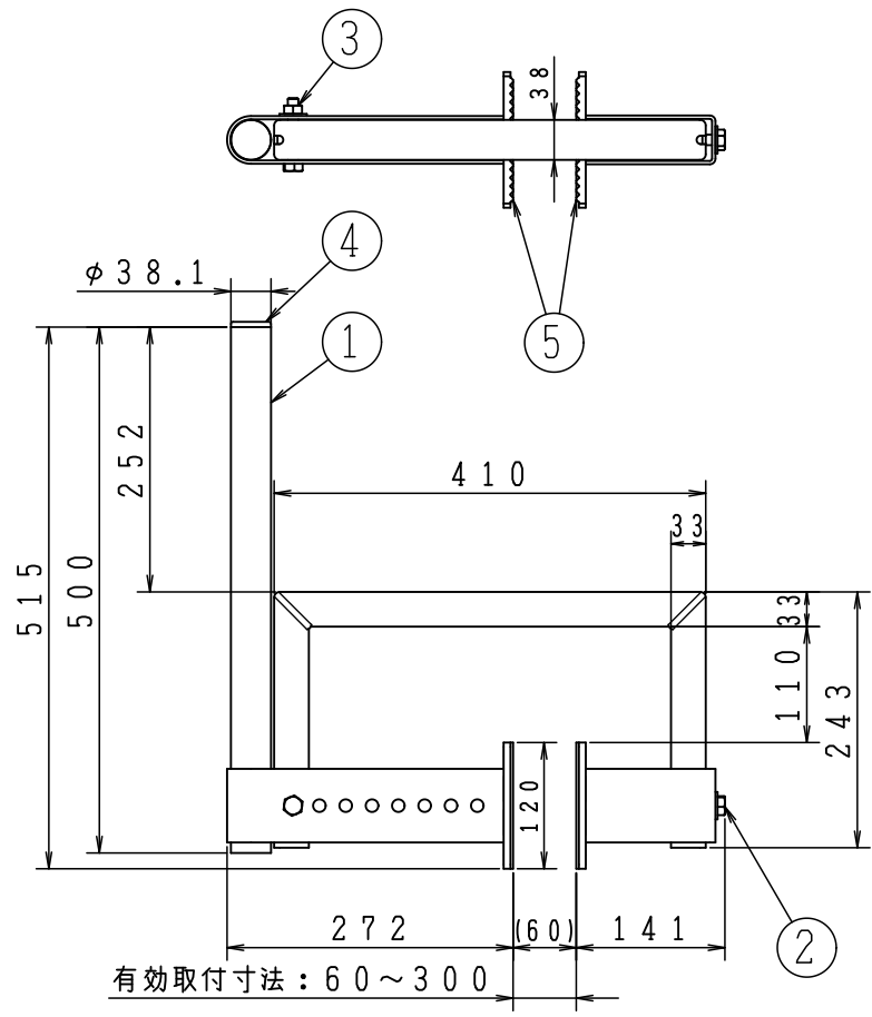
【取付寸法 60 mm の場合】
